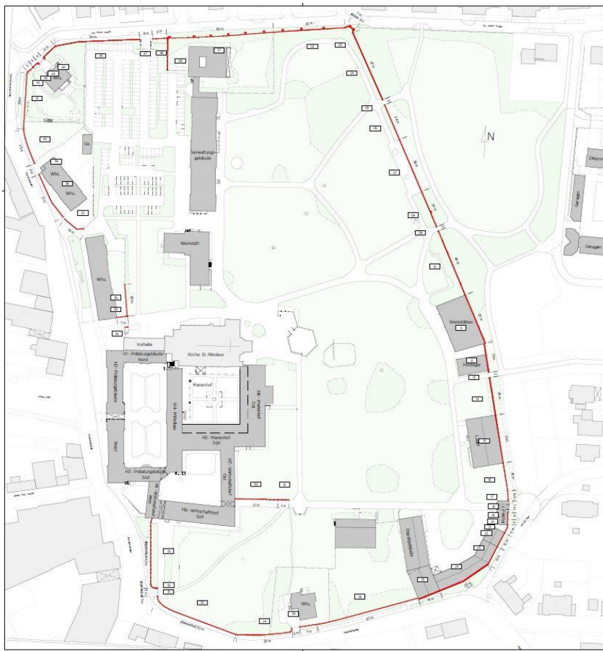
Lageplan Abtei Brauweiler mit Immunitätsmauer
