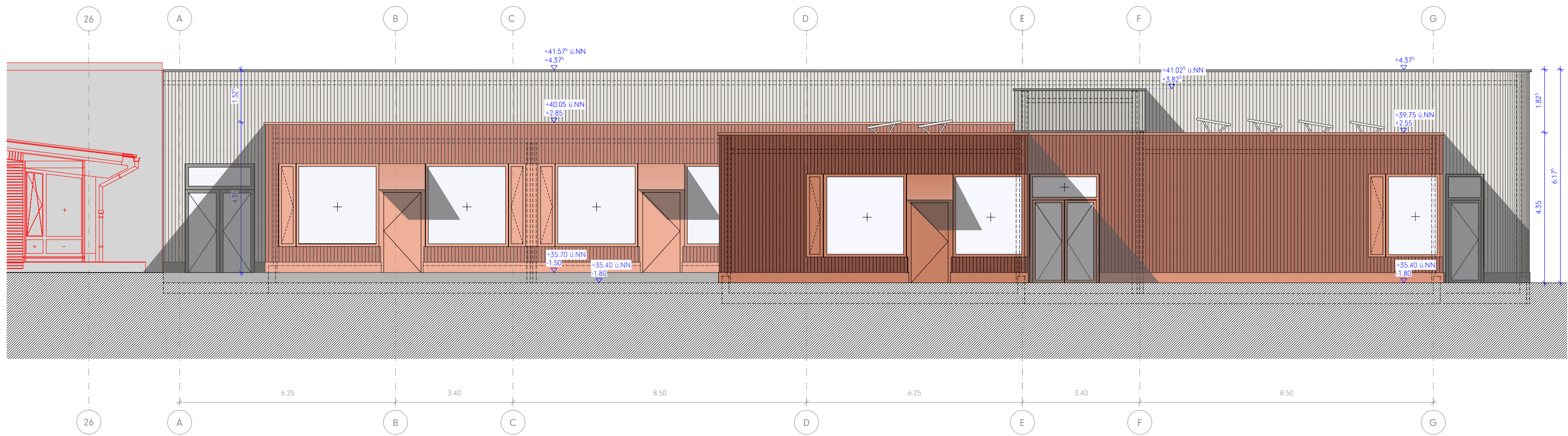
Ansicht West
